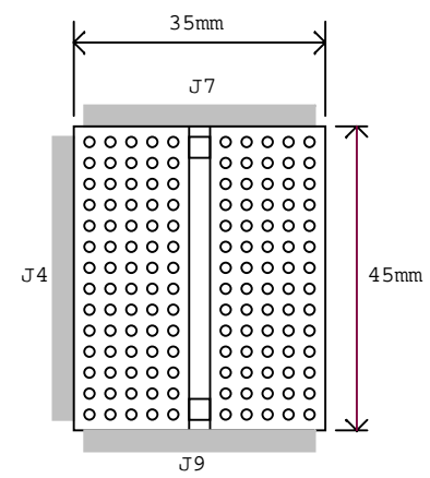
브레드 보드(Bread Board)
